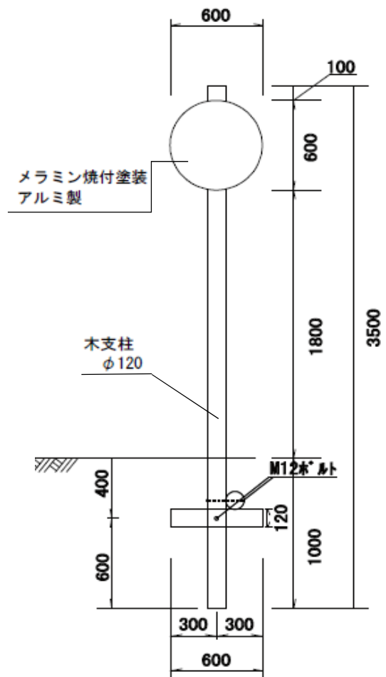
【側面図】
